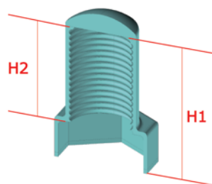
3D断面図
