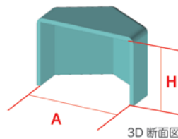
3D 断面図
