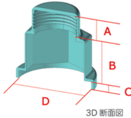
3D 断面図
