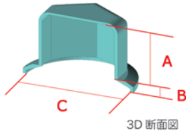
3D断面図
