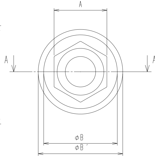
上面図
