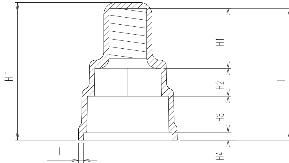
断面図
