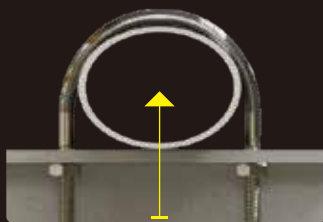
Uボルトの締め付けすぎで鋼材が変形
