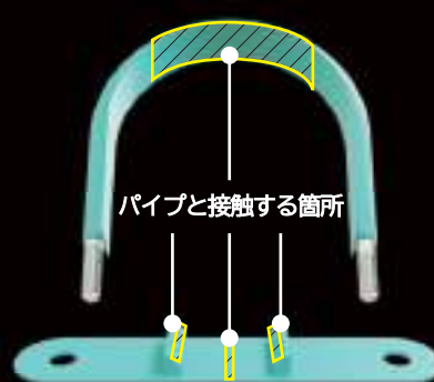
スタビプレート
